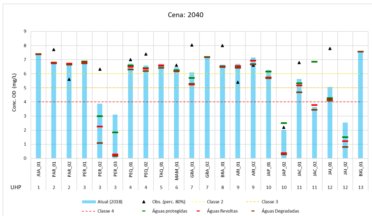
Figura 10.12 – Resultados das simulações de qualidade da água nos Pontos de Controle para o cenário atual e os três cenários socioeconômicos para a cena de 2040 – Parâmetro: OD.
